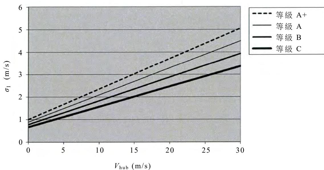
圖 1(a) 擾流強度標準差
