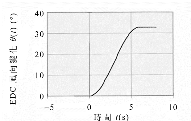
圖 4 極端風向暫態變化示例
