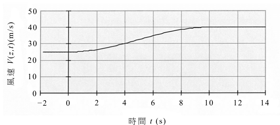
圖 5 ECD 極端相干陣風大小之示例
