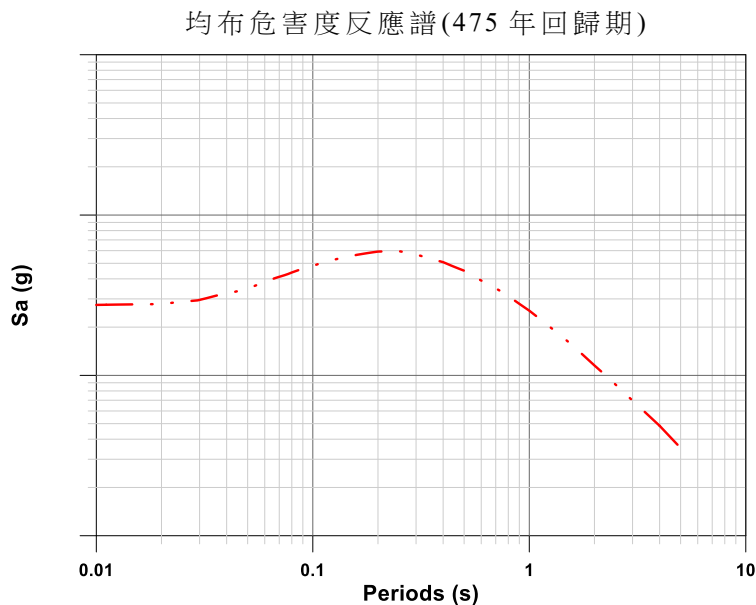
圖 I.2 風力機支撐結構之地震動反應譜(本圖僅為示意圖，不同場地情況不同)
