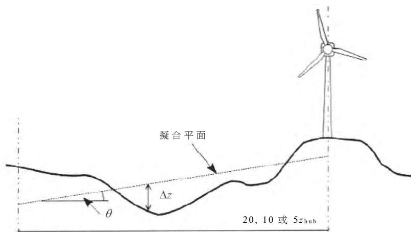
圖 10 用於擬合地形資料之 30^\circ 扇形區間示例
