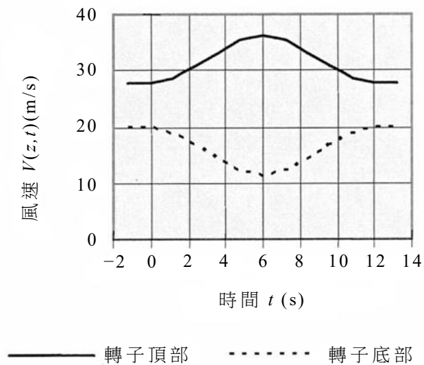
圖 9 轉子頂部與底部之風速示例，其顯示暫態正風切
