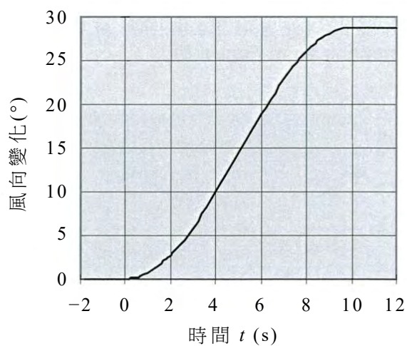
圖 7 暫態風向變化示例
