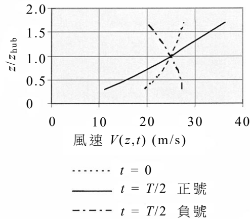
圖8 極端正及負垂直風切，開始時( t = 0 \text{ s} ，虛線)及最大風切時( t = 6 \text{ s} ，實線)之風剖面示例
